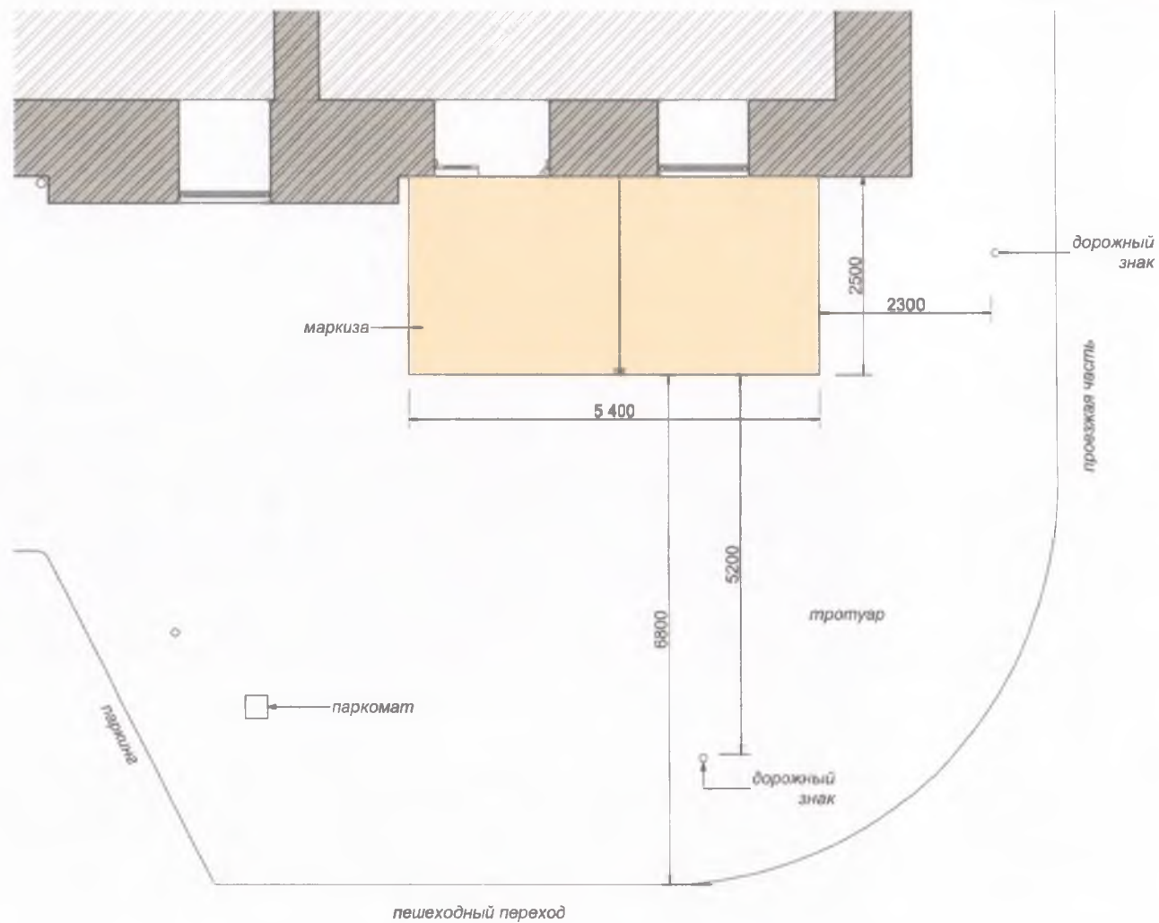
План размещения оборудования. М 1:80
